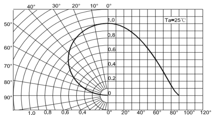
辐射图特性曲线
